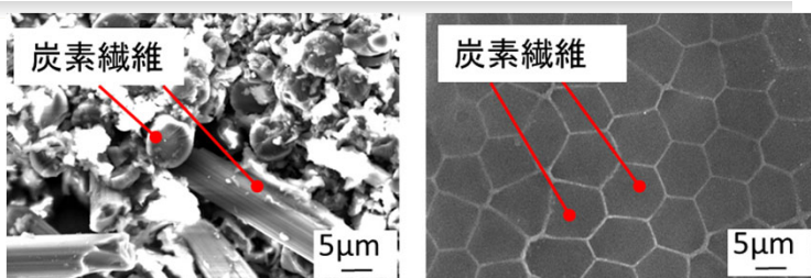
(a)切削加工面 (b)本研究における加工面 図 加工面の状態比較
